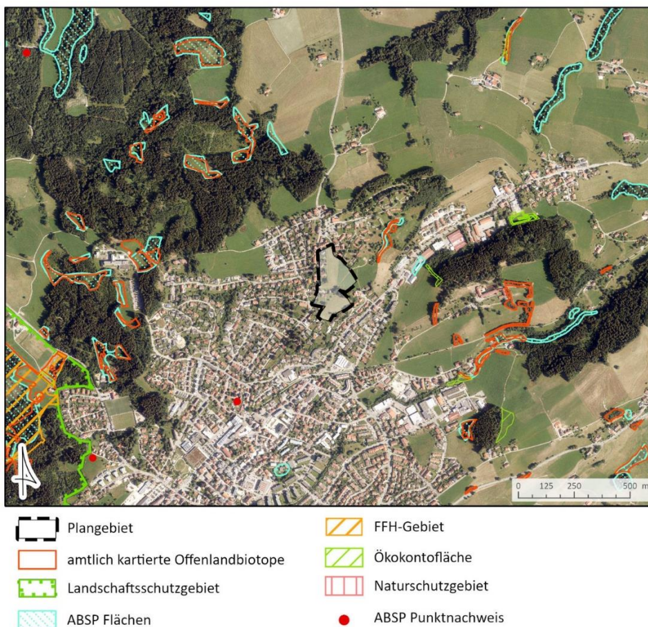
Abbildung 4: Schutzgebiete, amtlich kartierte Biotopie im Umfeld des Untersuchungsgebiets
