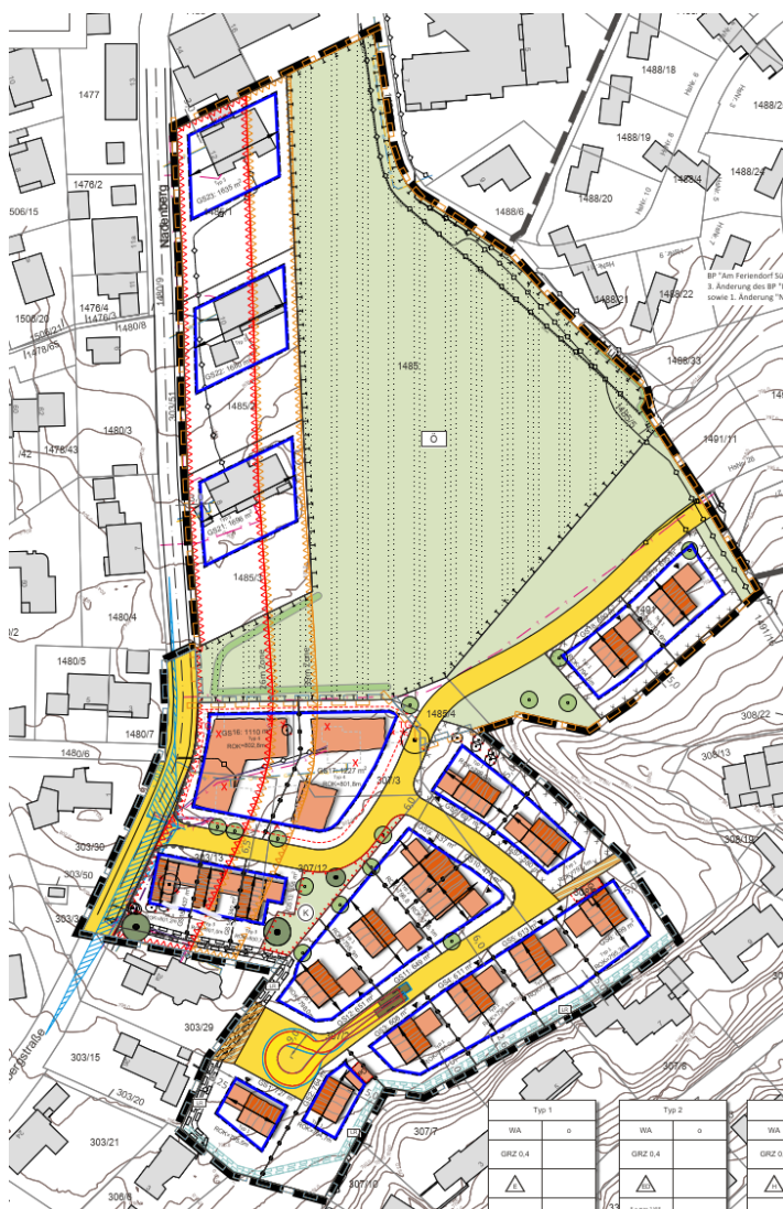
Abbildung 3: Bebauungsplan
